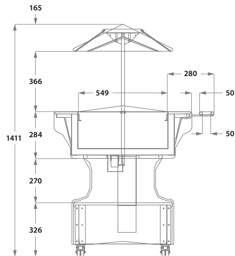
Seitenansicht Samoa 4/1 GN
