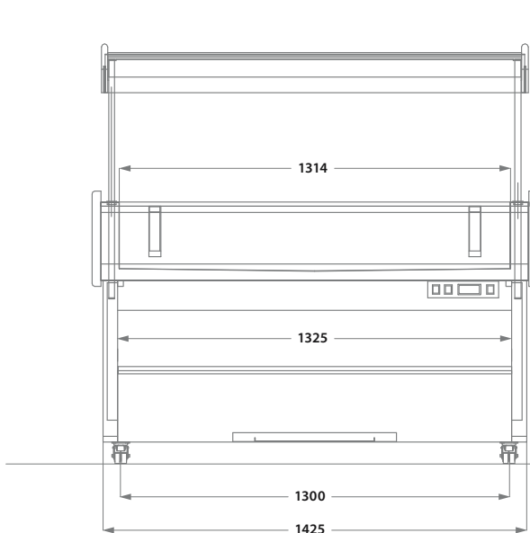
Frontansicht Samoa 4/1 GN
