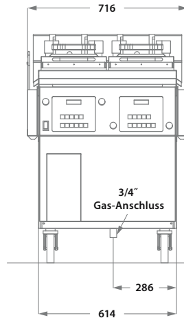
Frontansicht
