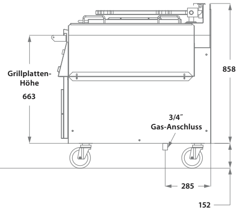
Seitenansicht rechts
