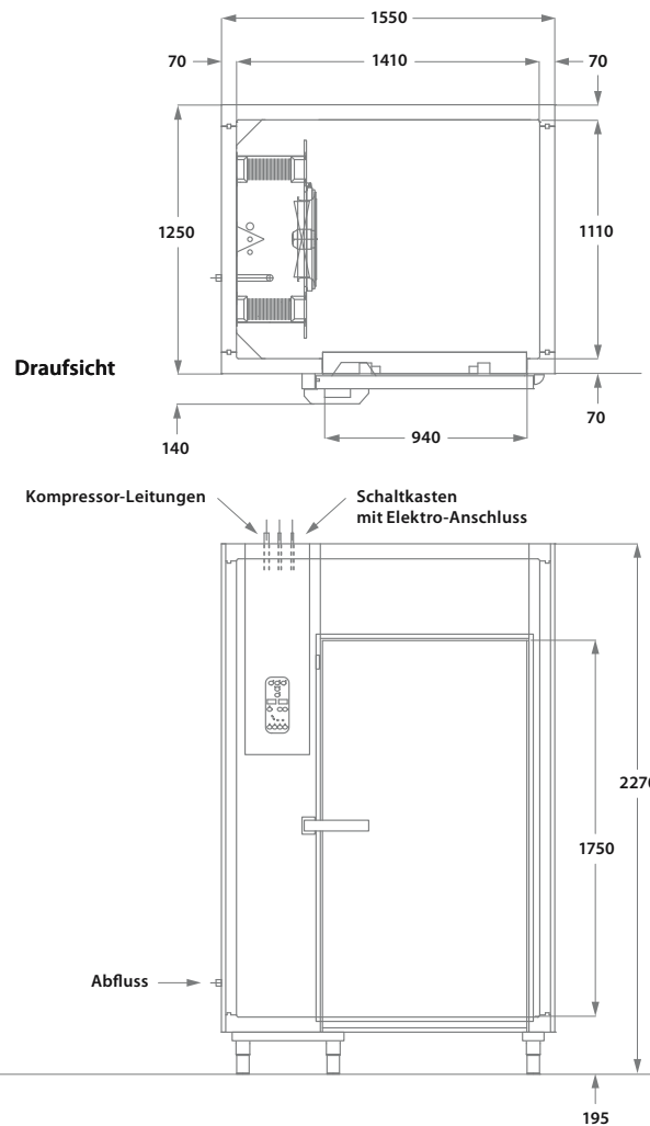
Frontansicht
