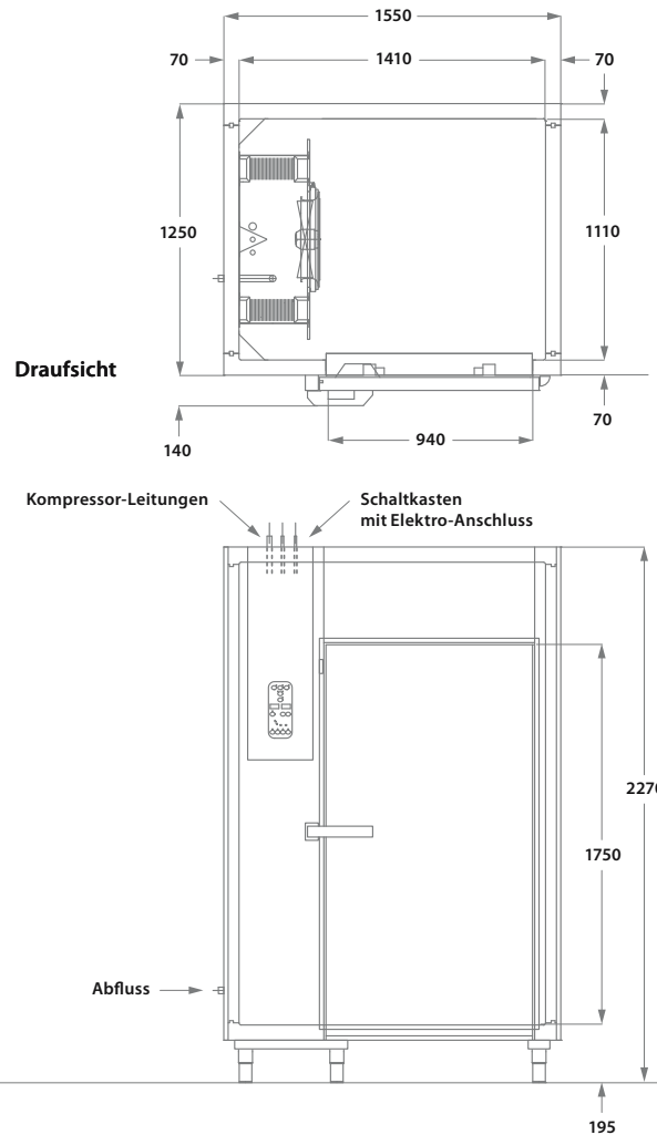
Frontansicht
