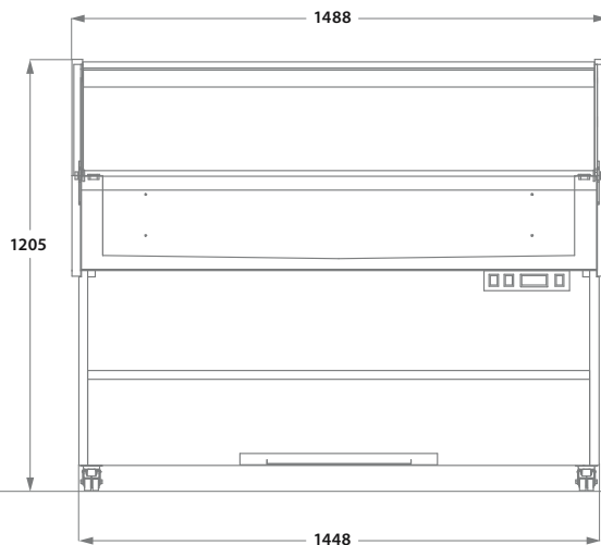
Frontansicht
