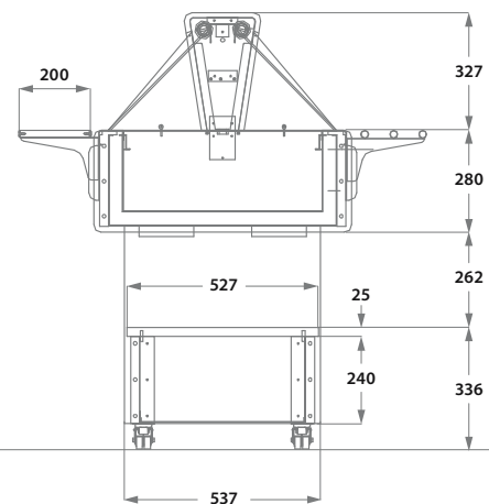
Seitenansicht
