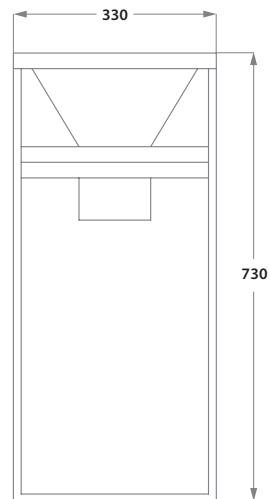
Seitenansicht
