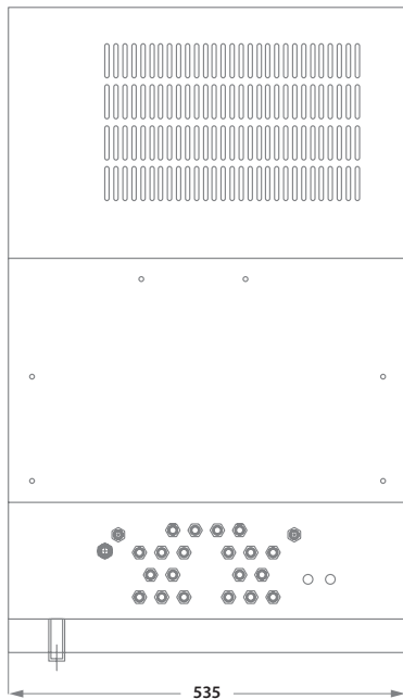
Draufsicht
